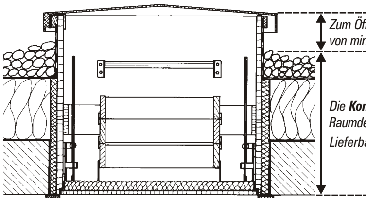
Zeichnung: Bodentreppe mit Zusatzausstattung FlachdachAusstieg
