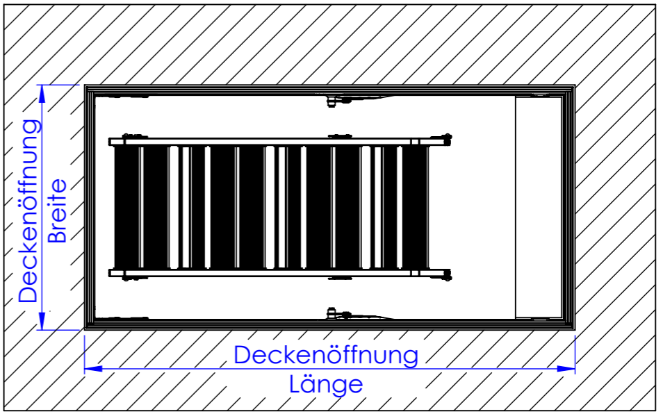
Deckenanschluss
