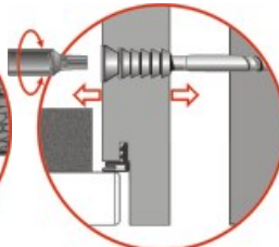
Justierschrauben
