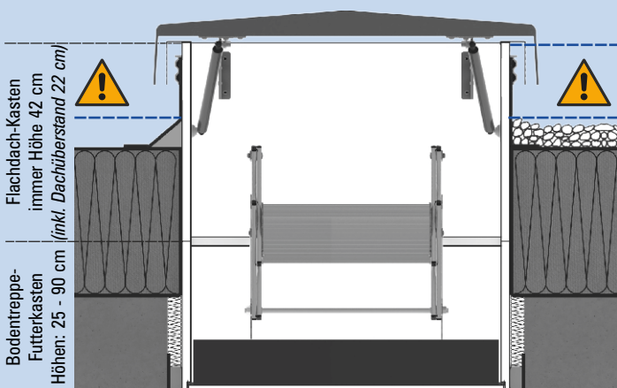
Abb.: FlachdachAusstieg mit Scherentreppe Liliput mit WärmeSchutz WS4D
